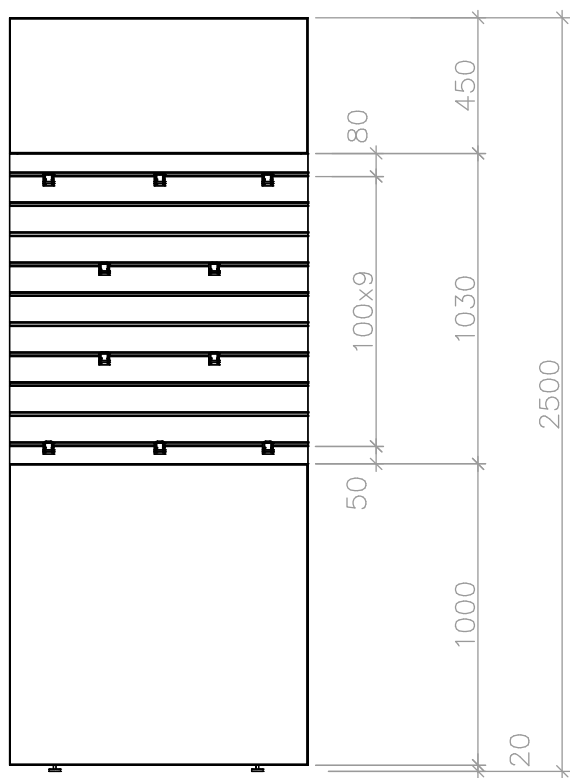
Ansicht Front/ Front view
